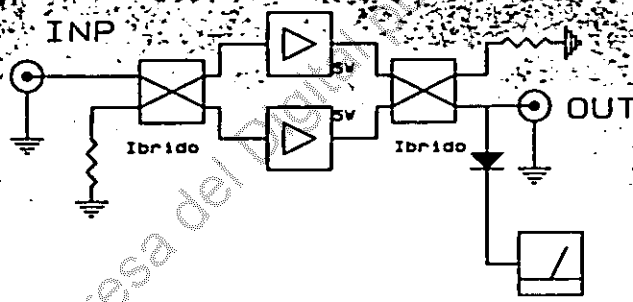
10 W AMPLIF.
