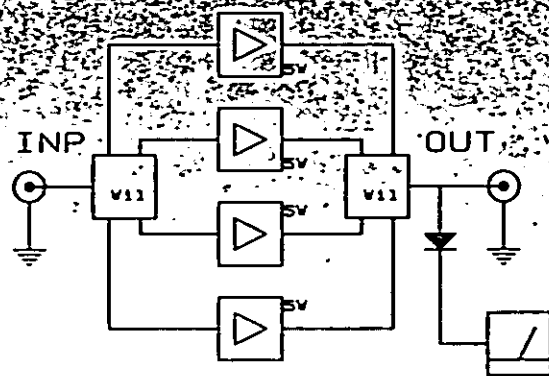
20 W AMPLIF.
