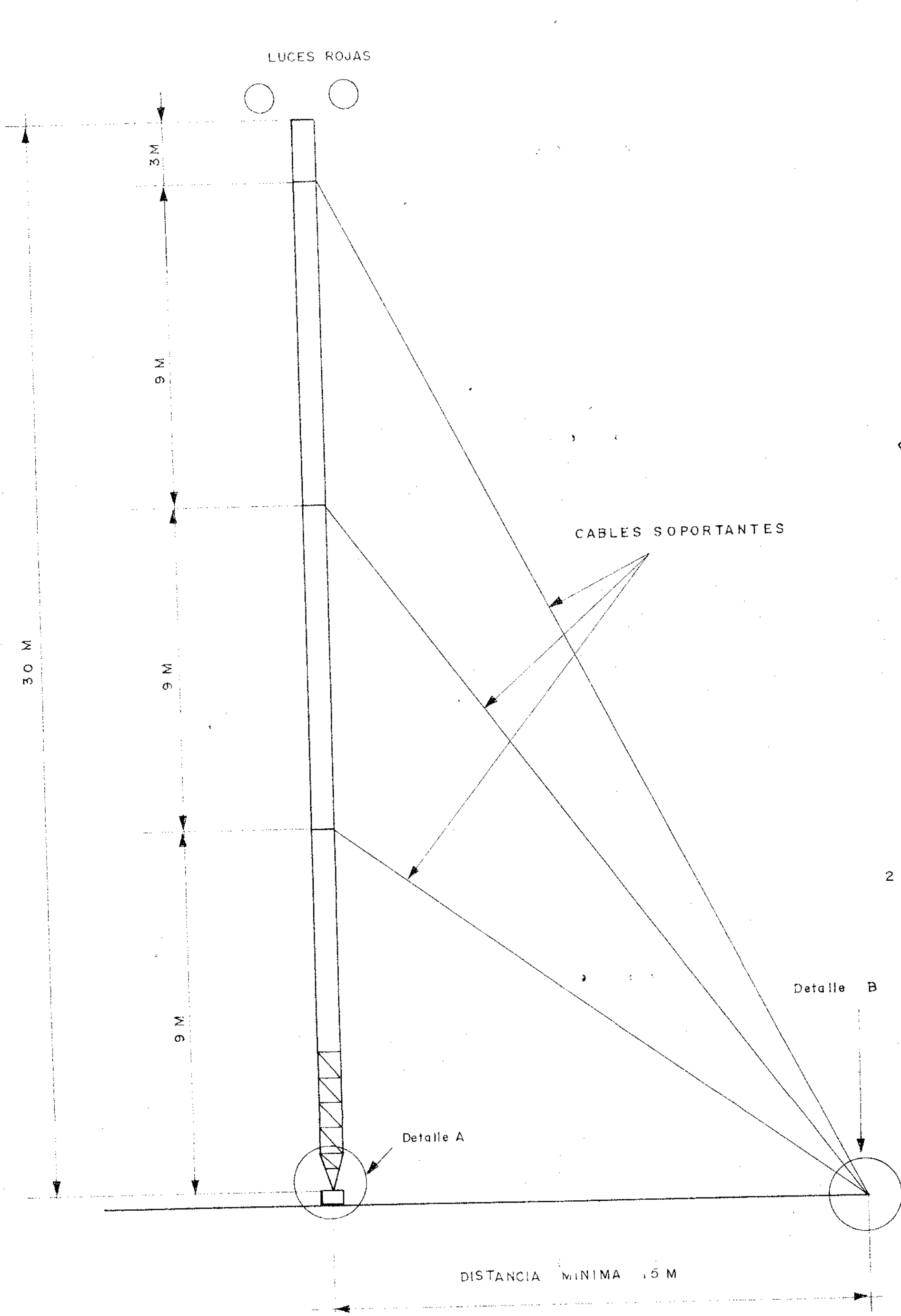
TORRE PARA REPETIDORA DE TV ESCALA 1/100
