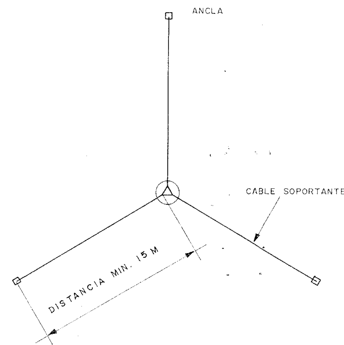
SISTEMA DE ANCLAJES ESCALA 1/200
