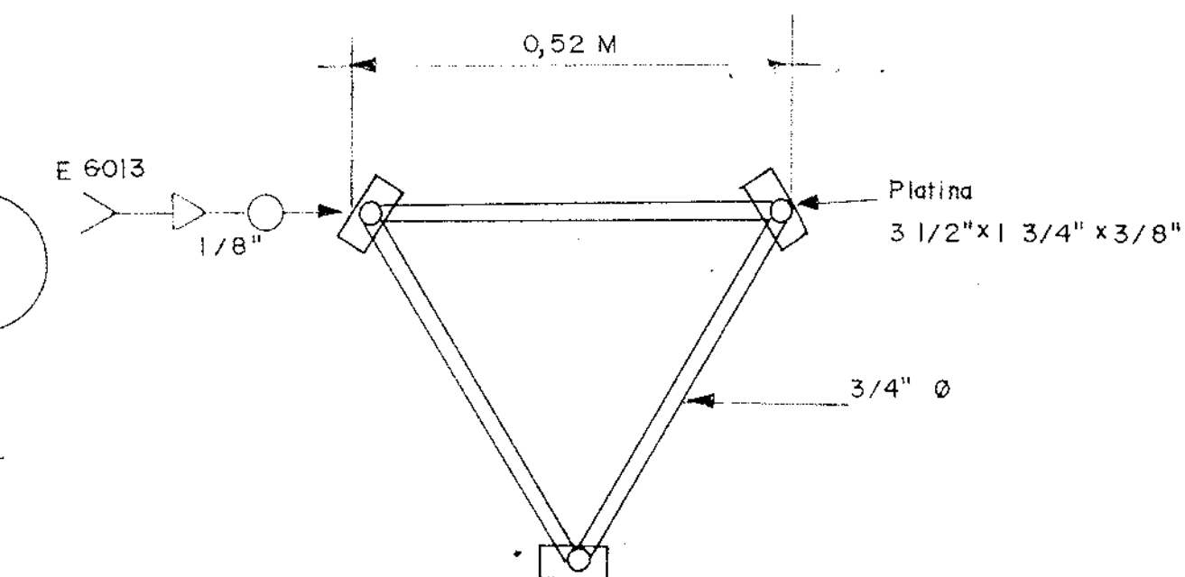
CORTE A-A ESCALA 1/8
