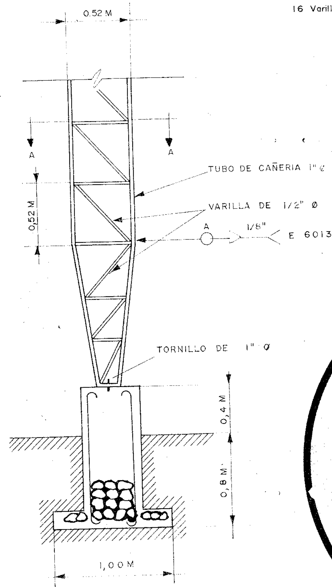
Detalle A ESCALA 1/20
