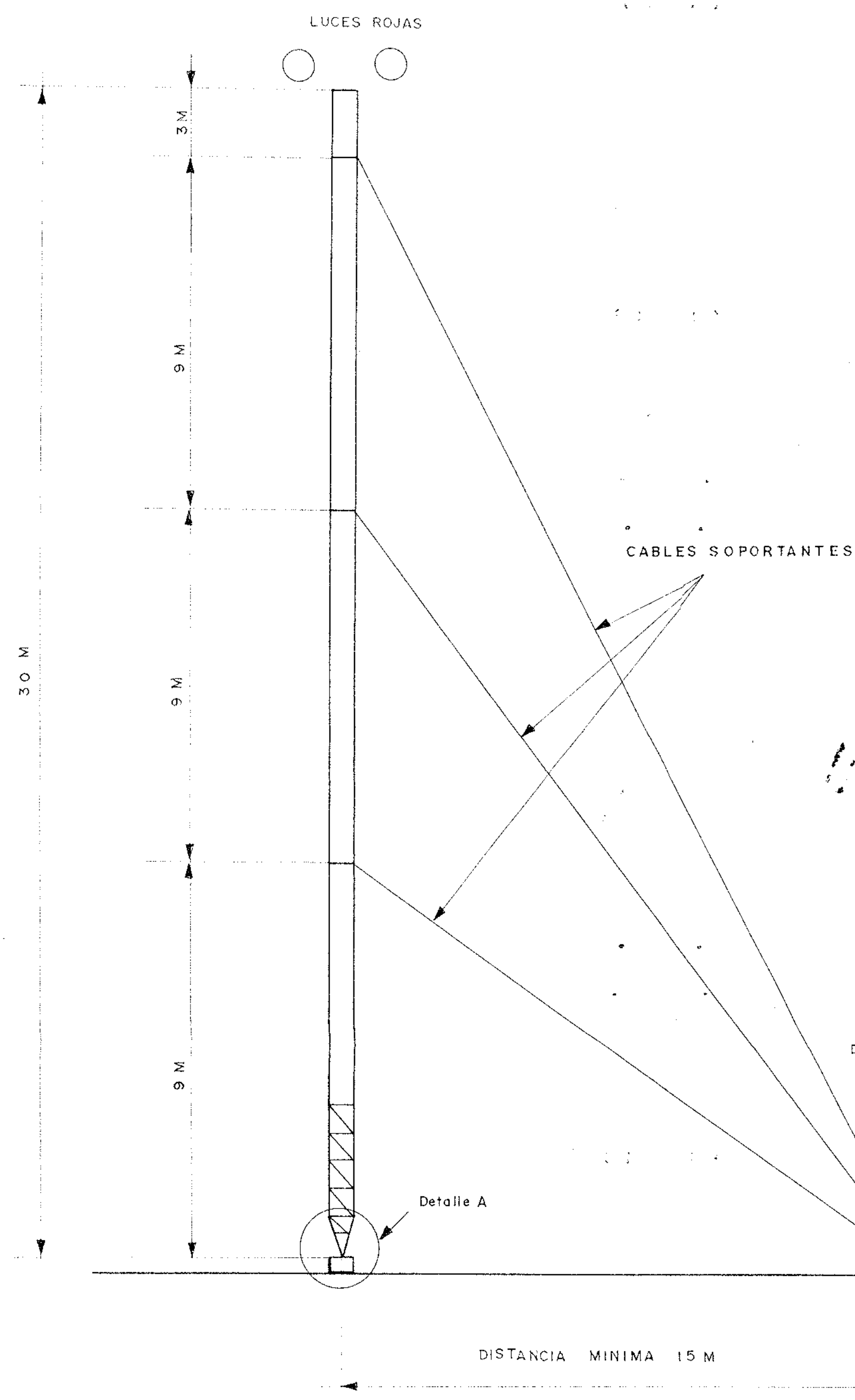
TORRE PARA REPETIDORA DE TV ESCALA 1/100
