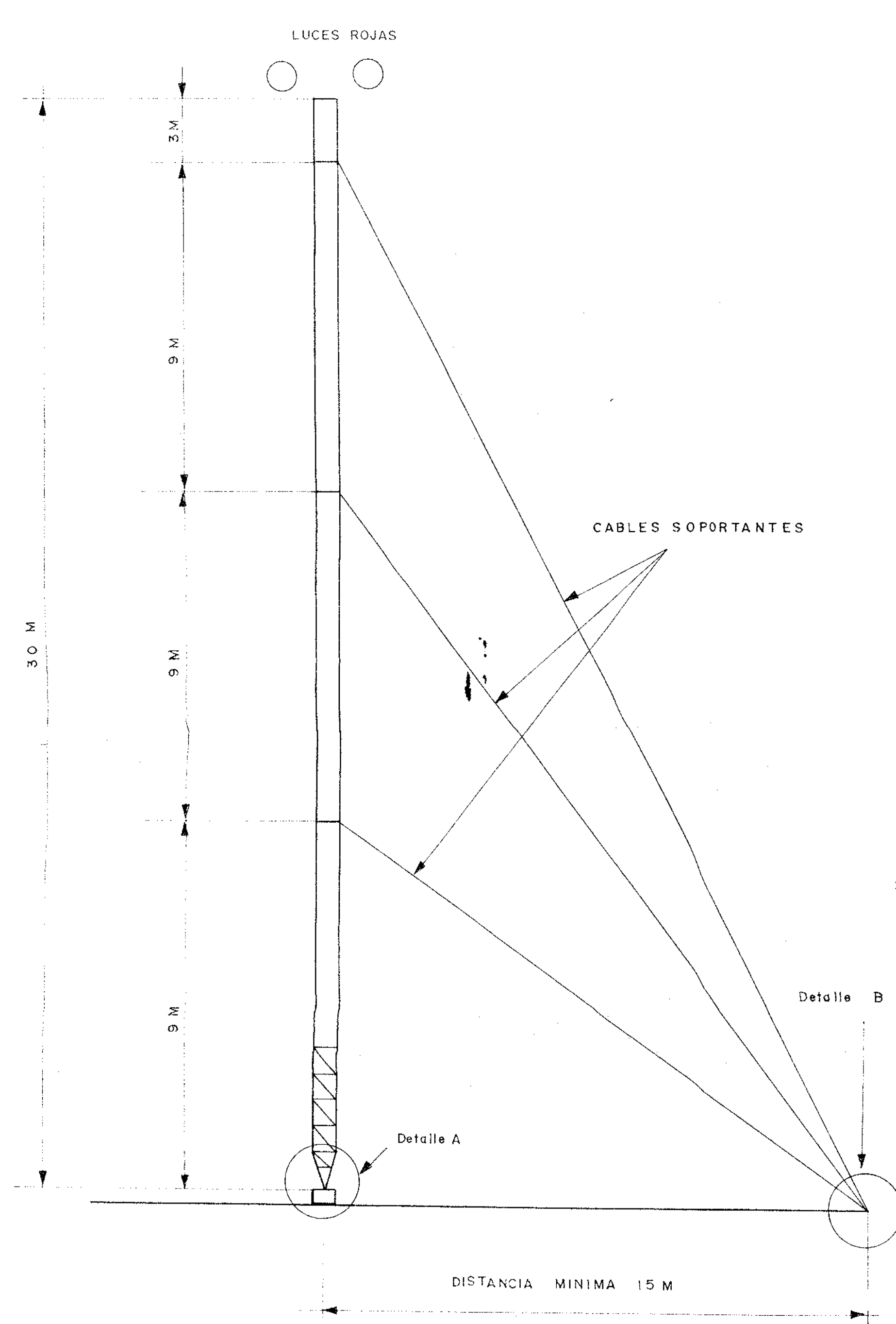
TORRE PARA REPETIDORA DE TV ESCALA 1/100
