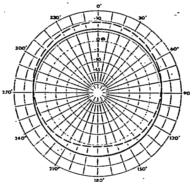
DB-224E (offset pattern)
