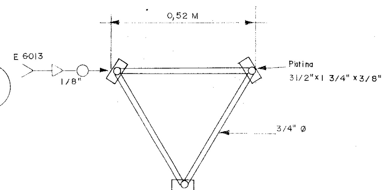
CORTE A-A ESCALA 1/8
